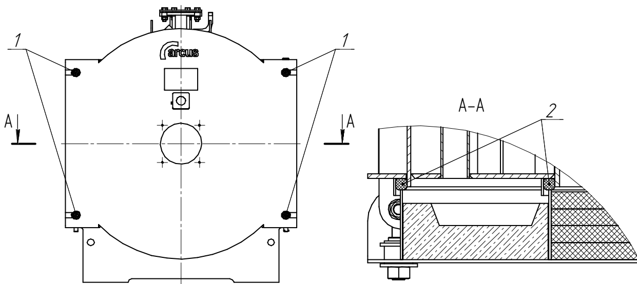
Рисунок 7. Передняя крышка.
