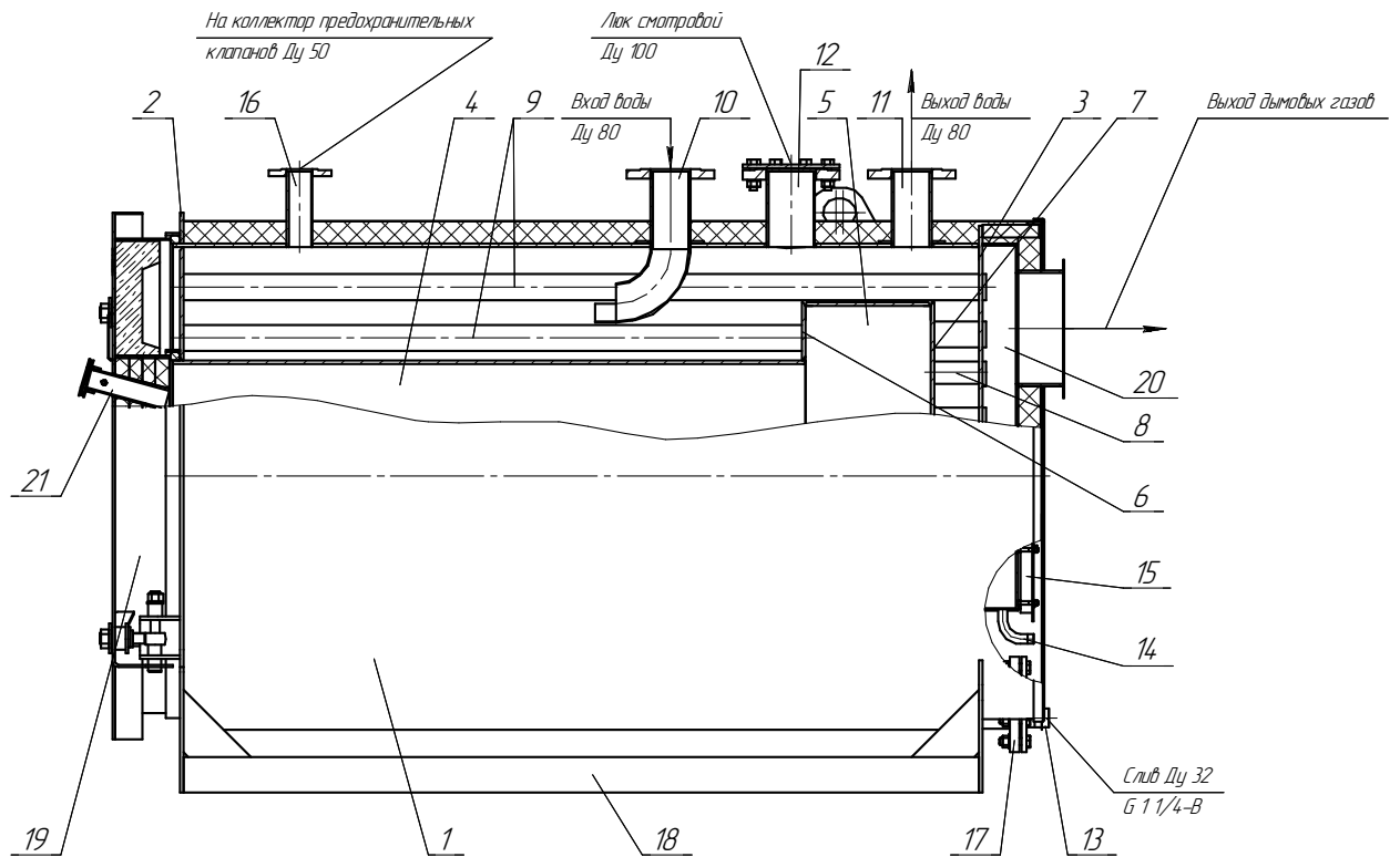
Рисунок 1. Схема котла
