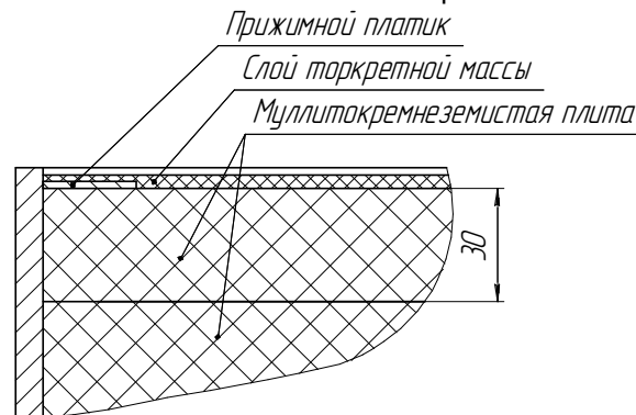
Рисунок 9. Разрез смотрового люка.
