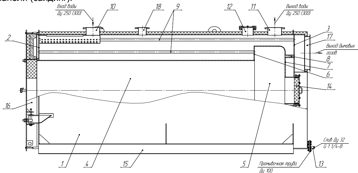
Рисунок 1. Схема котла
