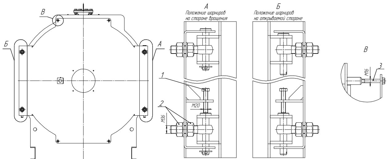
Рисунок 7. Передняя крышка.
