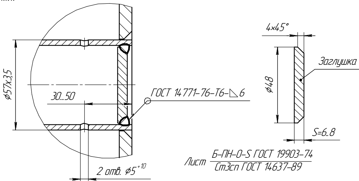
Рисунок 8. Установка заглушки.
